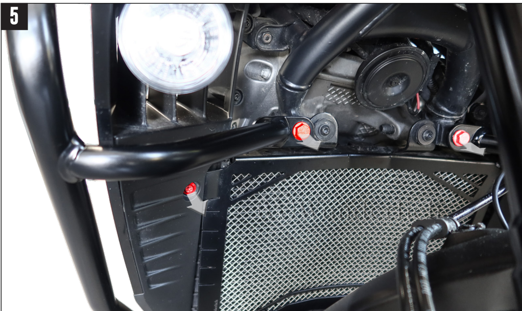
Microfloater und Halter vormontieren. Pre-assemble the Microfloater and bracket. Pré-assemblez le Microfloater et le support.
