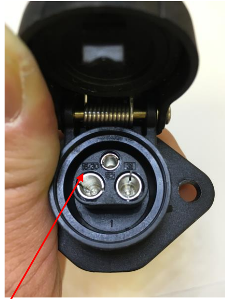
Frontansicht Kontakt „30“ Plus (+)
