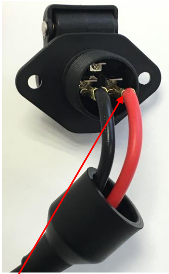
Von hinten, rechter Kontakt Plus (+), rotes Kabel
